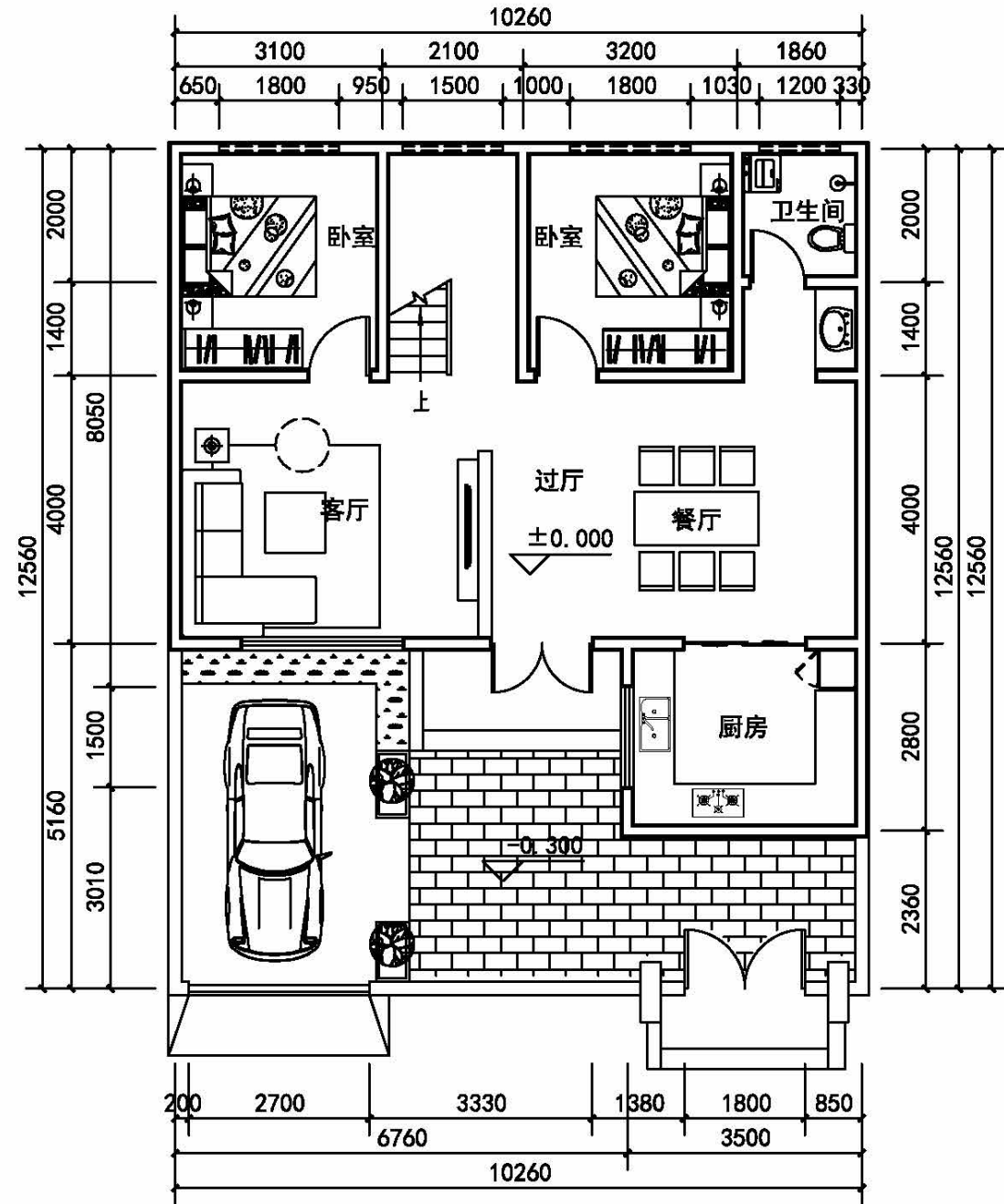
一层平面图 1:100
