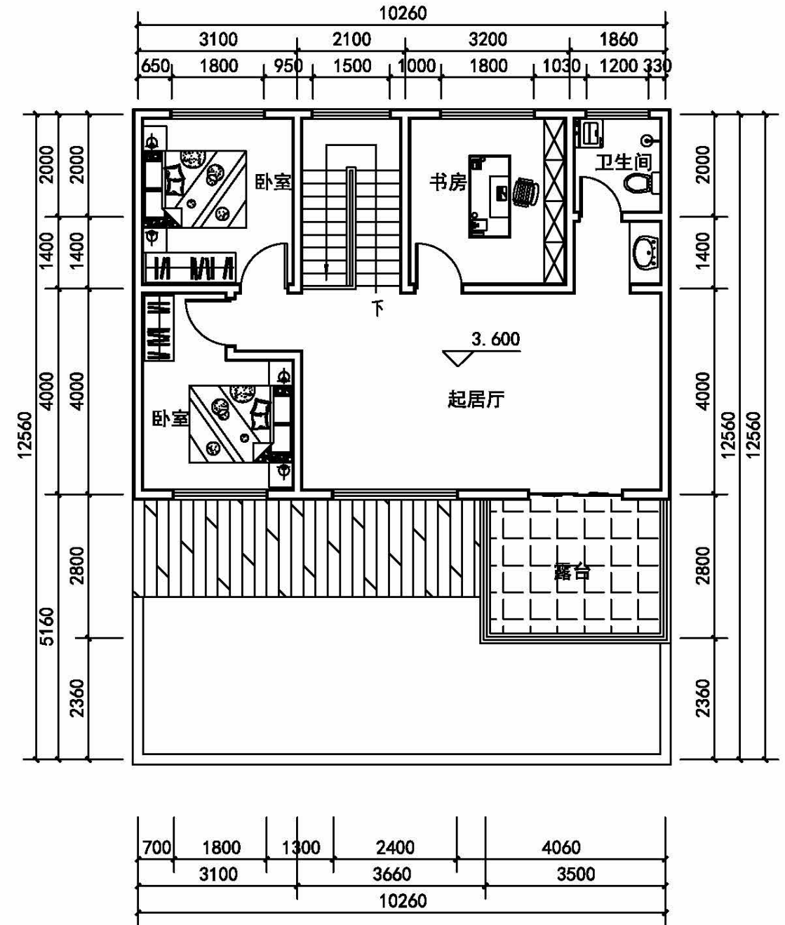
二层平面图 1:100
