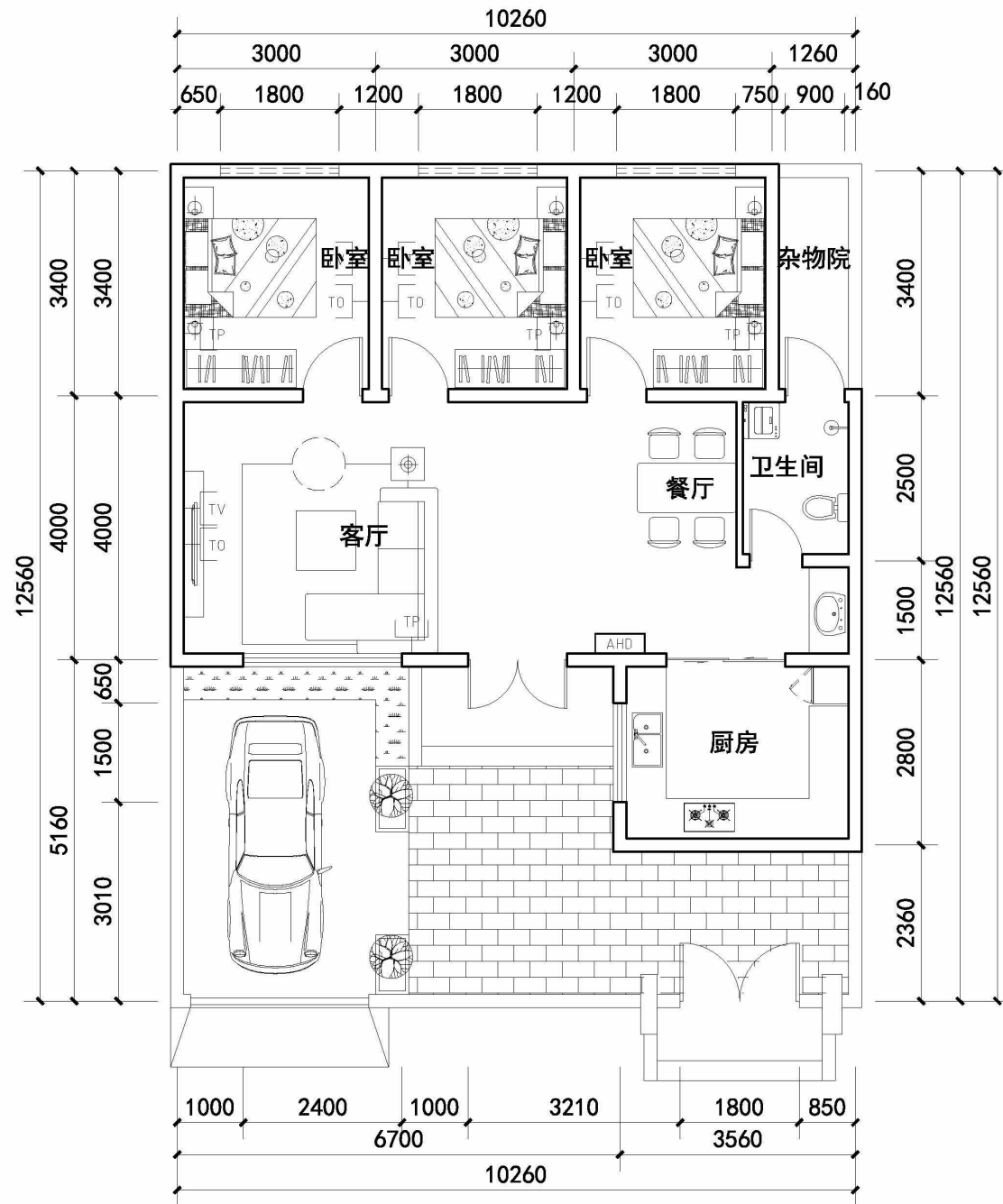
一层弱电平面图 1:100
